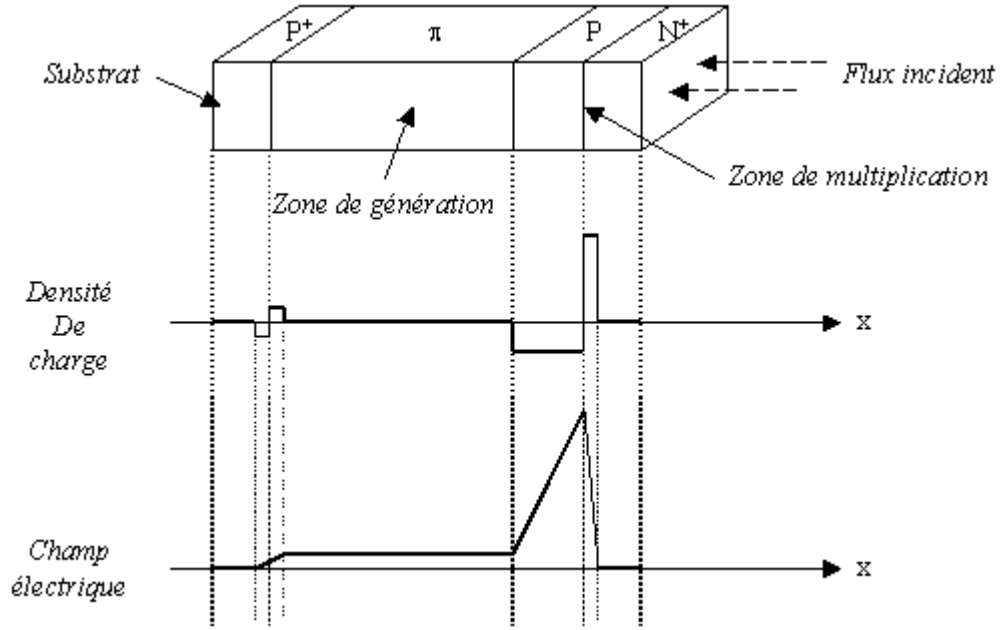
Figure II-g : Structure d'une photodiode à avalanche polarisée en inverse de manière à dépeupler totalement la zone P et la zone π. ( -400\text{ V} < V_{APD} < -150\text{ V} pour le silicium).
