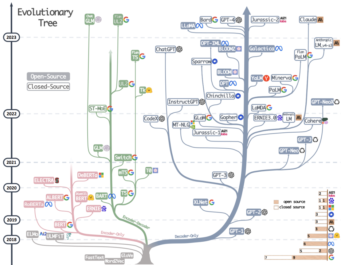
FIGURE 2.17 – Arbre du développement LLMs de 2018 à 2023. On observe à partir de 2022 une forte croissance du nombre de modèles développés pour l'analyse de texte basés sur les architectures de transformers . (J. YANG et al., 2023)
