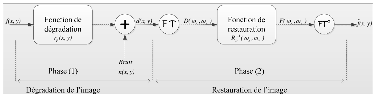
Fig. IV.1 : Un modèle du processus dégradation/restauration de l'image.
