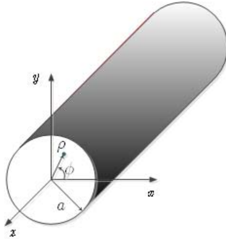
Fig. III.9: Guide d'onde cylindrique ouvert.
