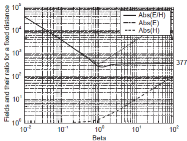
Fig. I.11 : Les modules des champs E , H , et du rapport E/H en fonction de \beta à une distance fixe r=1
