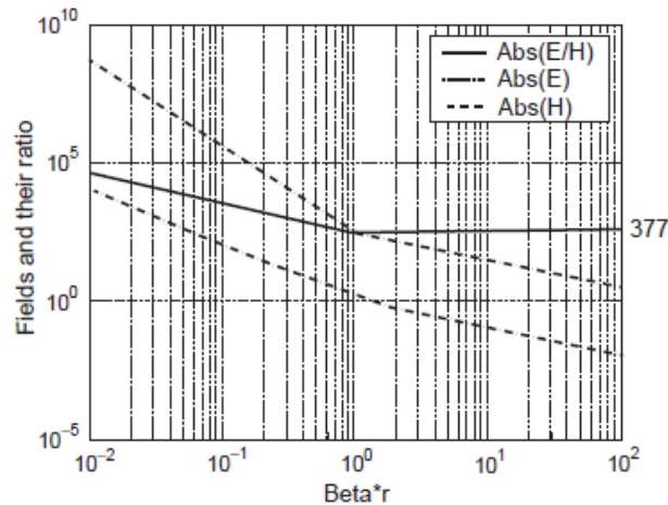
Fig. I.10 : Les modules des champs E , H , et du rapport E/H en fonction de (\beta.r) à une fréquence fixe
