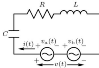
Figure 2.32: Modélisation d'un inducteur dans le cas d'un RLC série [33]
