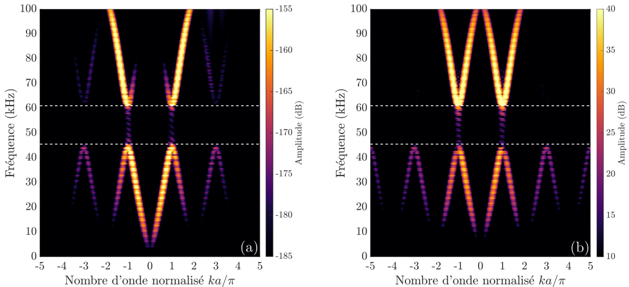
FIGURE 2.41 – Courbes de dispersion issues de simulations avec une électrode sur 5 reliée à une masse commune à travers une résistance R_{min} = 1 \text{ }\Omega . Le graphique (a) correspond à la double transformée de Fourier du champ de déplacement fenêtré et le (b) à celle du relevé fenêtré des potentiels électriques.
