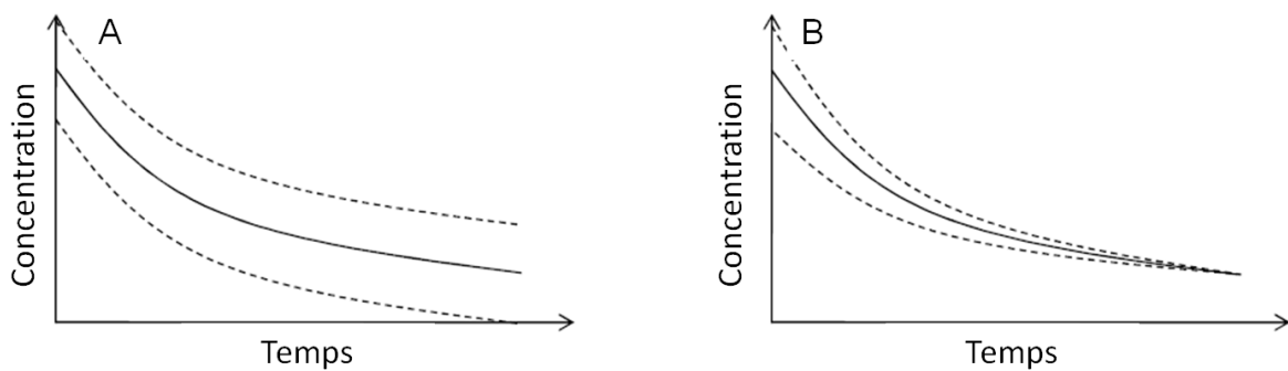
Figure 7 : Modèles d'erreur
