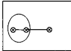
FIGURE 7.17 – Diagramme mal formé parce que deux croix reliées sont dans la même région minimale, d'après Shin 1994, p. 62
