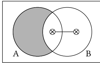
FIGURE 9.1 – Exemple de diagramme de Shin-Venn
