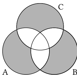
FIGURE 10.5 – Un autre diagramme de Venn symétrique par permutation de A, B, C
