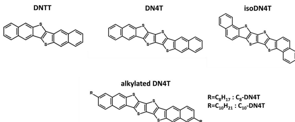
Figure R.1: Structures moléculaires du DNTT, DN4T, isoDN4T et des dérivés alkylés du DN4T.
