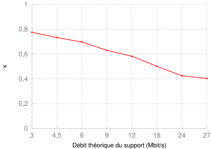
FIGURE 4.6 – \kappa en fonction du débit ( C ), la taille du fichier est de 1KB
