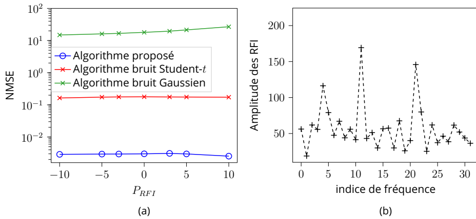
Figure 3.3 – Évolution du NMSE de \mathcal{Z} en fonction de la puissance des RFI de forte puissance en présence de RFI additionnelles de faible puissance sur chaque canal fréquentiel.
