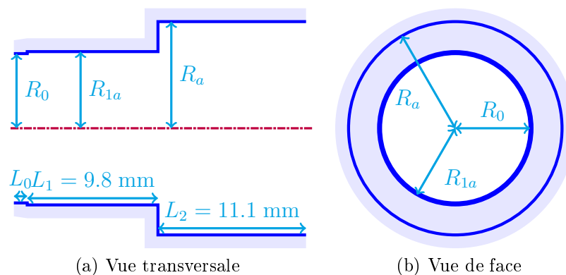
FIGURE 2.23 – Schéma d’une ouverture rayonnante à deux étages (échelle 2.5 :1) - R_a = 8 mm, R_{1a} = 5.75 mm.
