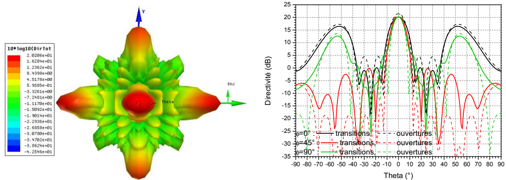
(a) Vue 3D de la directivité d'un panneau rayonnant avec HFSS. (b) Comparaison de la directivité pour le réseau excité directement par rapport au réseau excité par les transitions avec compensation des phases.
