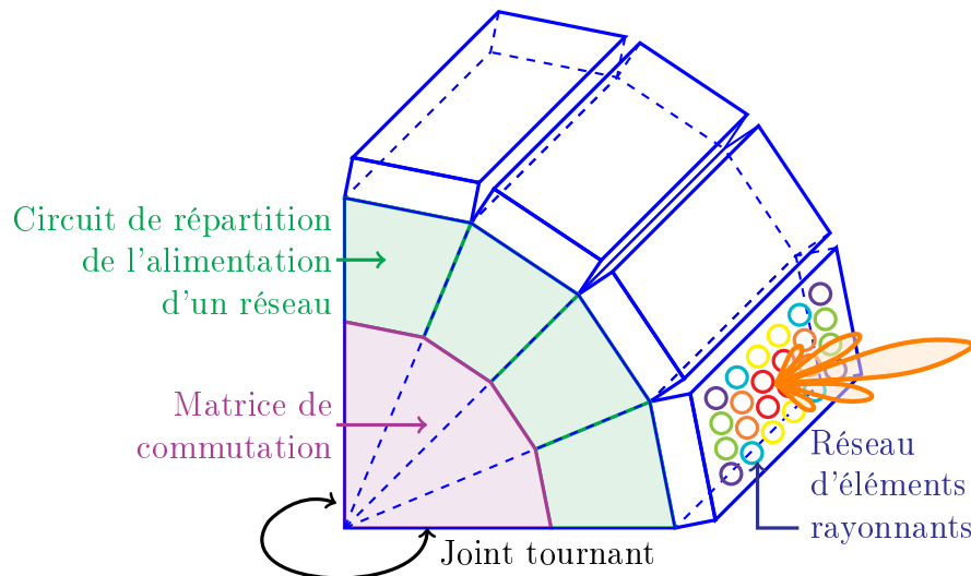
FIGURE 3.1 – Schéma de l'apparence générale du système antenneaire.
