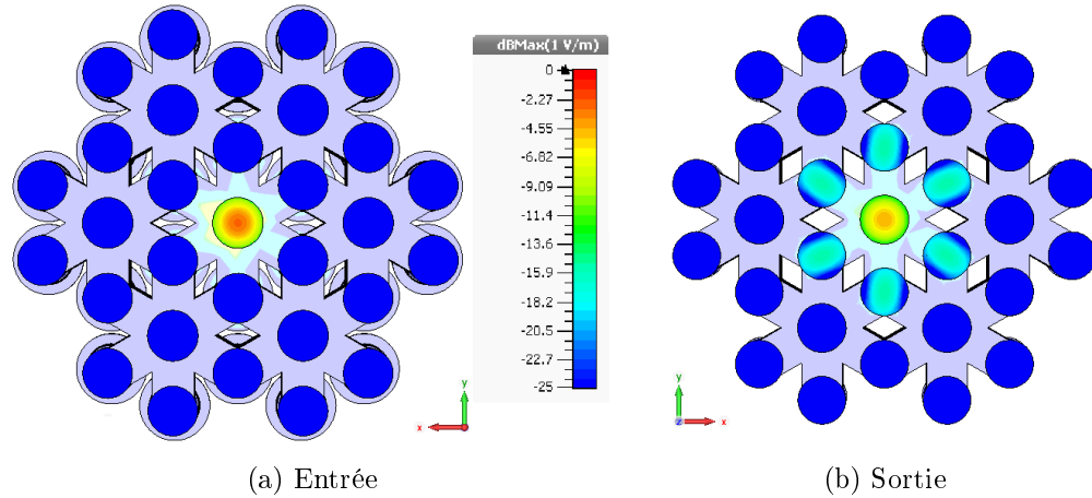
FIGURE 2.18 – Répartition de l'amplitude du champ électrique (a) en entrée et (b) en sortie des coupleurs en aluminium à 18.5 GHz pour une excitation en polarisation circulaire.
