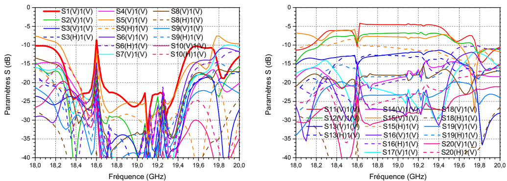
(a) Adaptation et paramètres S en isolation. (b) Paramètres S en transmission.
