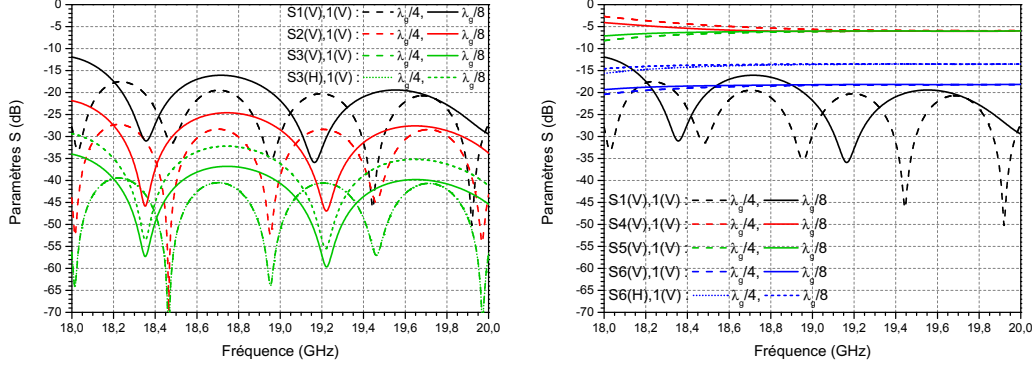
(a) Adaptation et paramètres S en isolation d'un coupleur en métal parfait. (b) Adaptation et paramètres S en transmission d'un coupleur en métal parfait.
