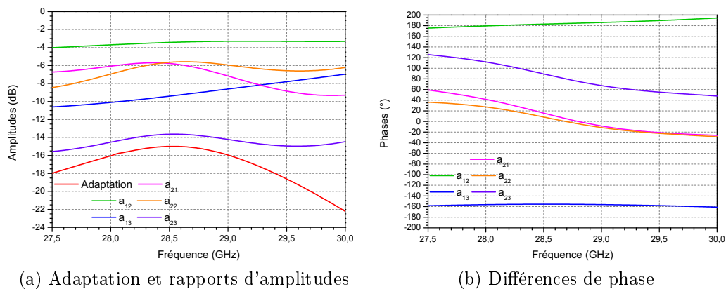
FIGURE 3.27 – Adaptation, rapports d'amplitudes et différences de phase pour le quart du circuit de répartition.
