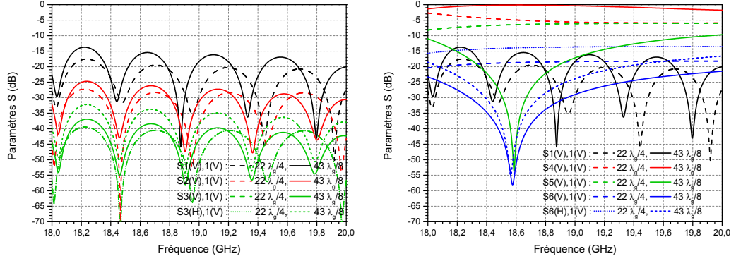
(a) Adaptation et paramètres S en isolation (b) Adaptation et paramètres S en transmission d'un coupleur en métal parfait.
