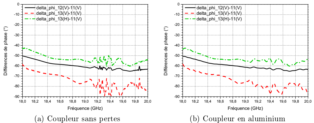
FIGURE 2.19 – Différence de phase entre les guides périphériques et le guide central en sortie des couplageurs (a) en métal parfait et (b) en aluminium pour une excitation en polarisation verticale.
