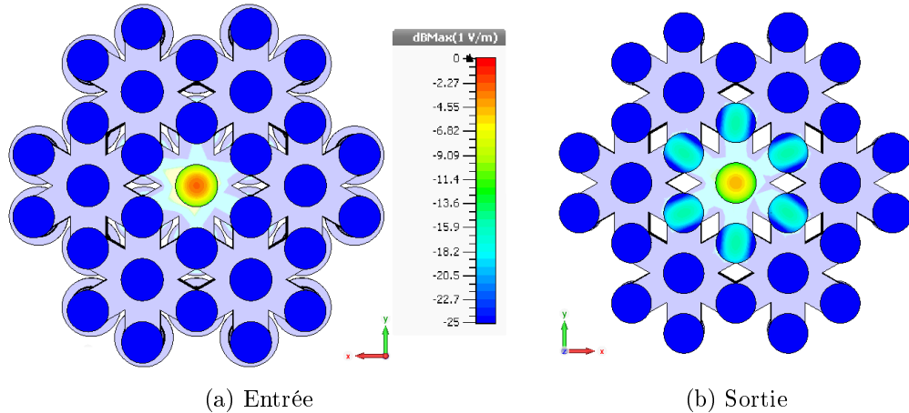
FIGURE 2.18 – Répartition de l'amplitude du champ électrique (a) en entrée et (b) en sortie des couplageurs en aluminium à 18.5 GHz pour une excitation en polarisation circulaire.
