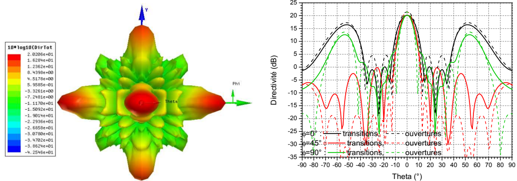
(a) Vue 3D de la directivité d'un panneau rayonnant avec HFSS.
