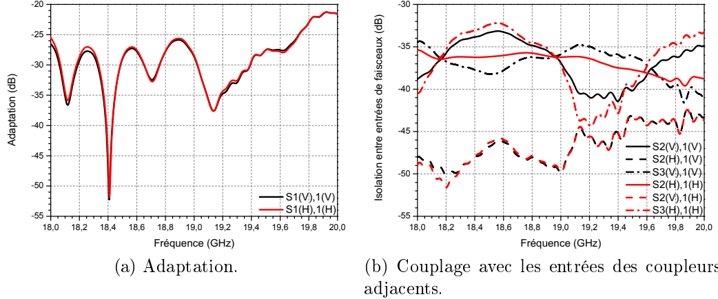
FIGURE 2.30 – (a) Adaptation et (b) couplage du réseau focal en aluminium simulé excité par une polarisation linéaire verticale puis horizontale.
