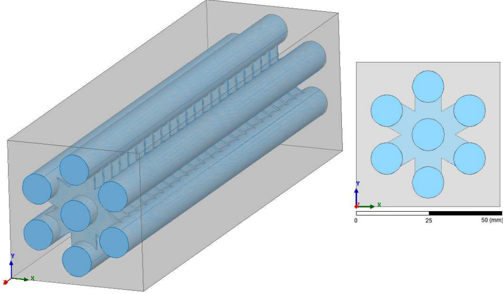
FIGURE 2.7 – Vues d'un coupleur.
