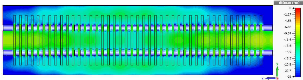
FIGURE 2.12 – Amplitude du champ électrique dans le plan x = 0 d'un coupleur à 43 fentes espacées de \lambda_g/8 .
