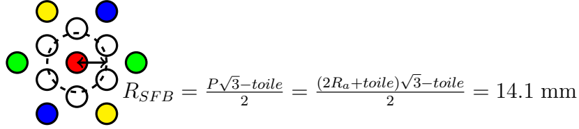
FIGURE 2.34 – Illustration d'un réseau d'éléments de type SFB dans la maille utilisée type MFB où 7 éléments rayonnants forment 1 faisceau. R_a = 8.0 \text{ mm} est le rayon de l'ouverture rayonnante, toile = 0.6 \text{ mm} est la partie métallique entre deux ouvertures.
