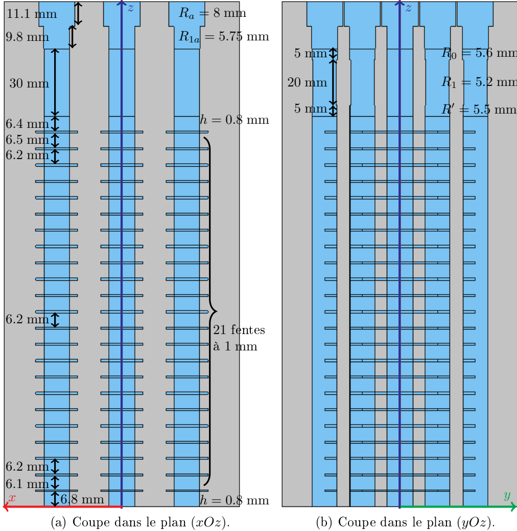
FIGURE 2.29 – Vues longitudinales de la source focale.
