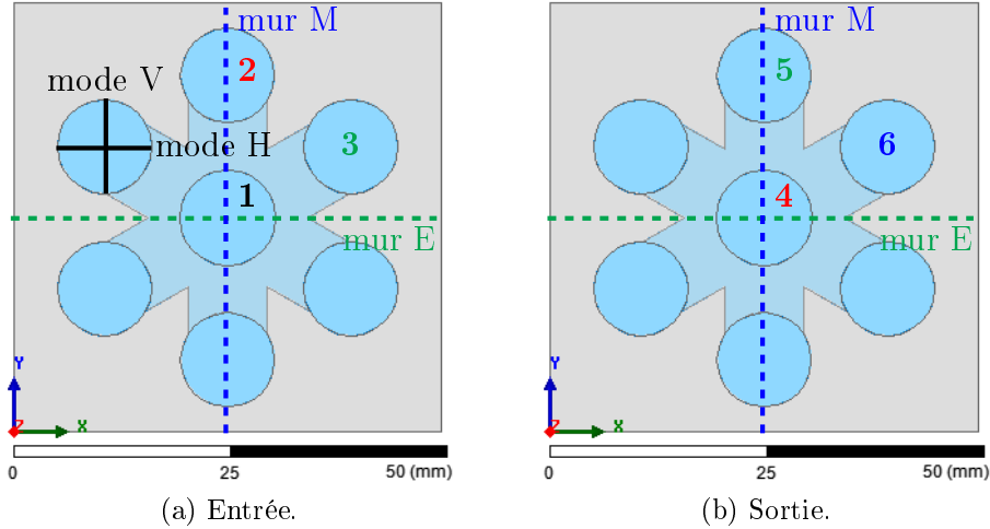
FIGURE 2.9 – Mise en évidence des plans de symétrie sur un seul coupleur et numérotation des ports.
