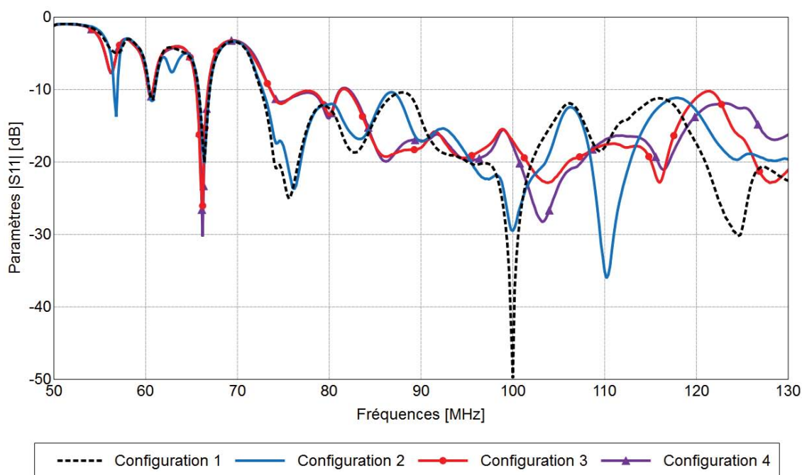
Figure 154 : Coefficient de réflexion en entrée de l'antenne VHF sur [50MHz ; 130MHz], Mesures en configurations n°1,2,3&4, H=32cm
