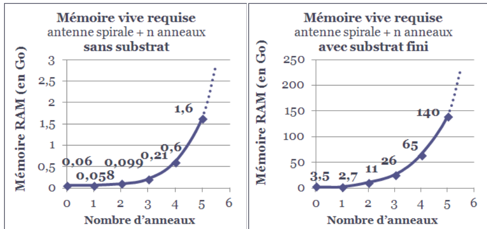
Figure 75 : Mémoire RAM nécessaire pour la simulation d'une antenne Ø1m sans puis avec substrat en fonction du nombre d'anneaux*
