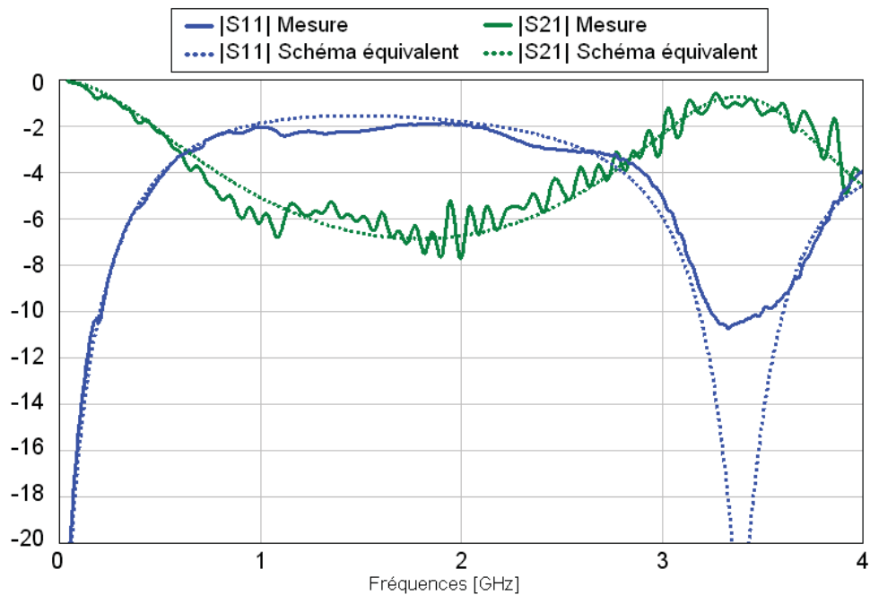
Figure 145 : Comparatifs Mesures-Schéma équivalent des paramètres |S_{11}| et |S_{21}| des deux câbles coaxiaux "back-to-back" pour la mesure des antennes VHF de Ø1m.
