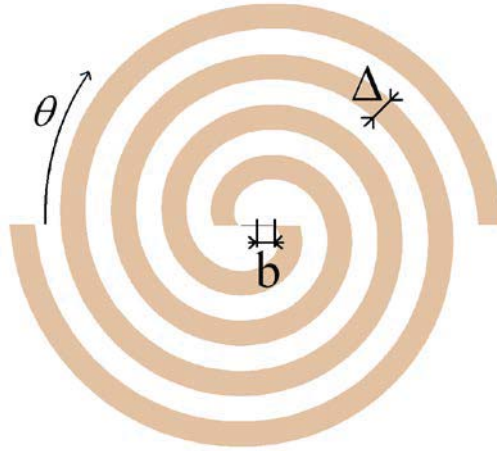
Figure 4 : Antenne spirale d'Archimède à deux brins
