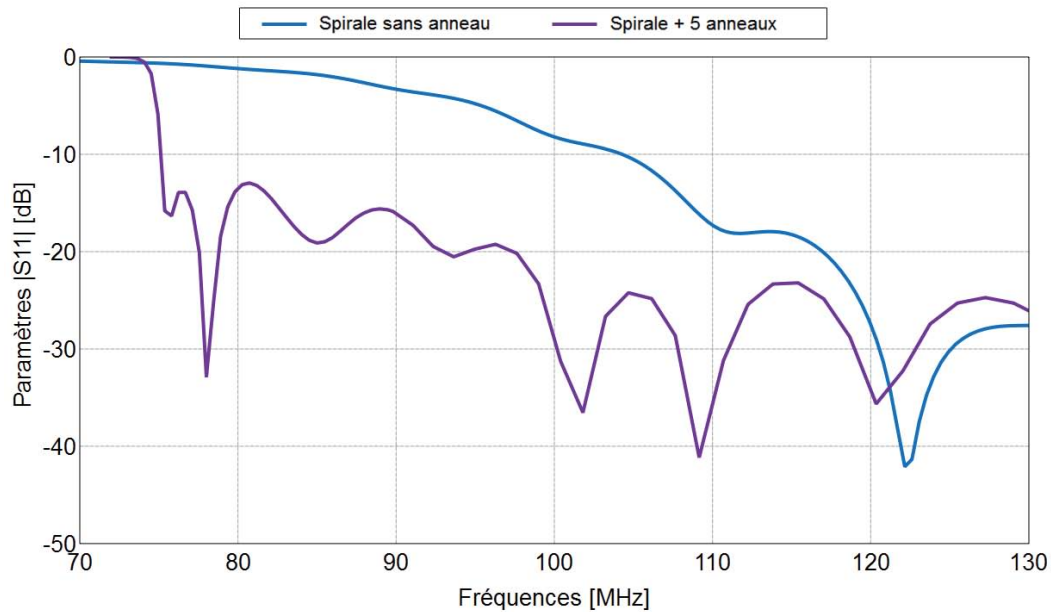
Figure 135 : Coefficient de réflexion en entrée des antennes spirales (Ø1m) à 0 et 5 anneau(x) sans substrat
