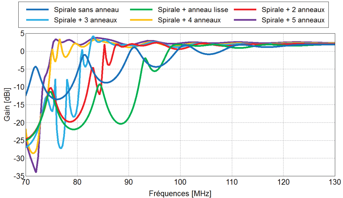
Figure 79 : Gain en polarisation principale (droite), en \theta=0^\circ , des antennes spirales ( \varnothing 1m ) + 0 à 5 anneau(x) sans substrat
