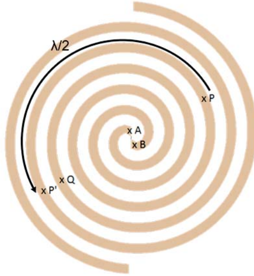
Figure 3 : Spirale d'Archimède
