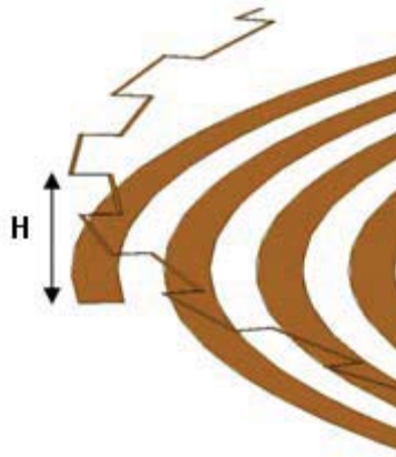
Figure 47 : Antenne spirale d'Archimède superposé d'un anneau crénelé
