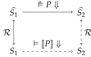
FIGURE 4.1 – Diagramme de commutation d’une propriété de préservation sémantique. Les flèches en trait plein représentent les relations en hypothèse de la propriété, tandis que celles en pointillés représentent les relations obtenues en conclusion.
