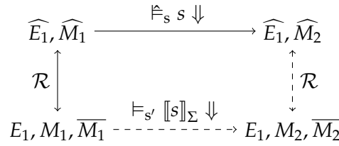
FIGURE 4.2 – Diagramme de commutation adapté aux langages d'étude.
