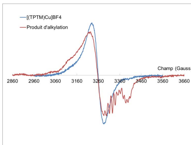
Figure 15 : Spectres RPE de [(\text{TPTM})\text{Cu}(\text{MeCN})]\text{BF}_4 et du produit de methylation (en solution dans le THF, 150K).
