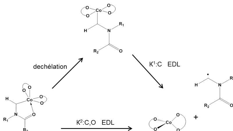
Schéma 8 : Procédés de déchélation et de rupture homolytique des liaisons de l'espèce dormante en Co-MRP des amides de vinyle avec le [\text{Co}(\text{acac})_2] ( \text{O}=\text{O}=\text{acac} ).
