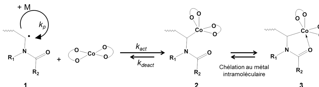
Schéma 7 : Equilibre de la Co-MRP d'amides de vinyle et phénomène de chélation sur le cobalt (acac = anion acétylacétonate).
