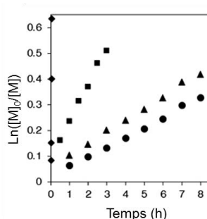
Figure 22 : \ln([M]_0/[M]) ( M = monomère) par rapport au temps de polymérisation pour la Co-MRP en masse de l'AcV (●), NVP (◆), NVCl (■), et NMVA (▲) amorcée à 40°C par un adduit cobalt-alkyle de faible masse molaire; [M]/[\text{Co}(\text{acac})_2(\text{PAcV})] = 380 (données issues de la référence 108).
