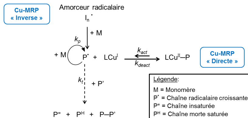
Schéma 5 : Mécanisme proposé de la polymérisation radicalaire contrôlée par le cuivre (Cu-MRP).
