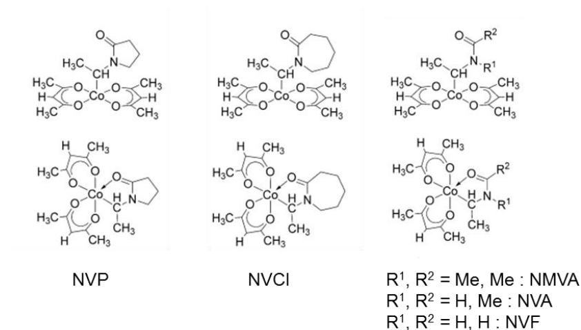
Figure 23 : Modèles des espèces dormantes de cobalt(III) penta- et hexa-coordiné pour la polymérisation des amides de vinyle.
