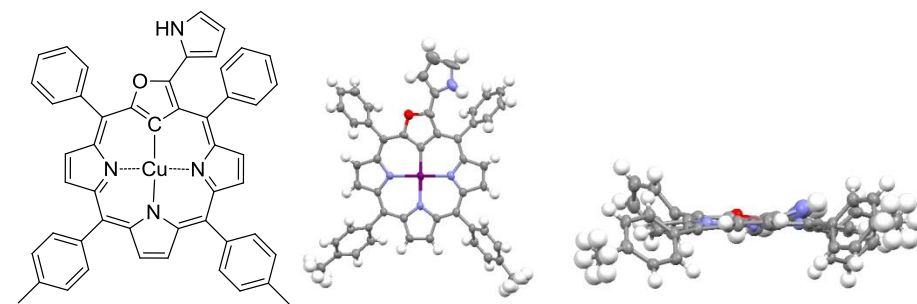
Figure 8 : Structure du complexe de cuivre(II) publiée par Latos-Grażyński 98 (représentation schématique; vue de haut et vue de côté de la structure RX). La distance Cu(II)-C est de 1.939(4) Å.
