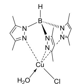
[\text{Tp}^*\text{CuCl}] hydraté
