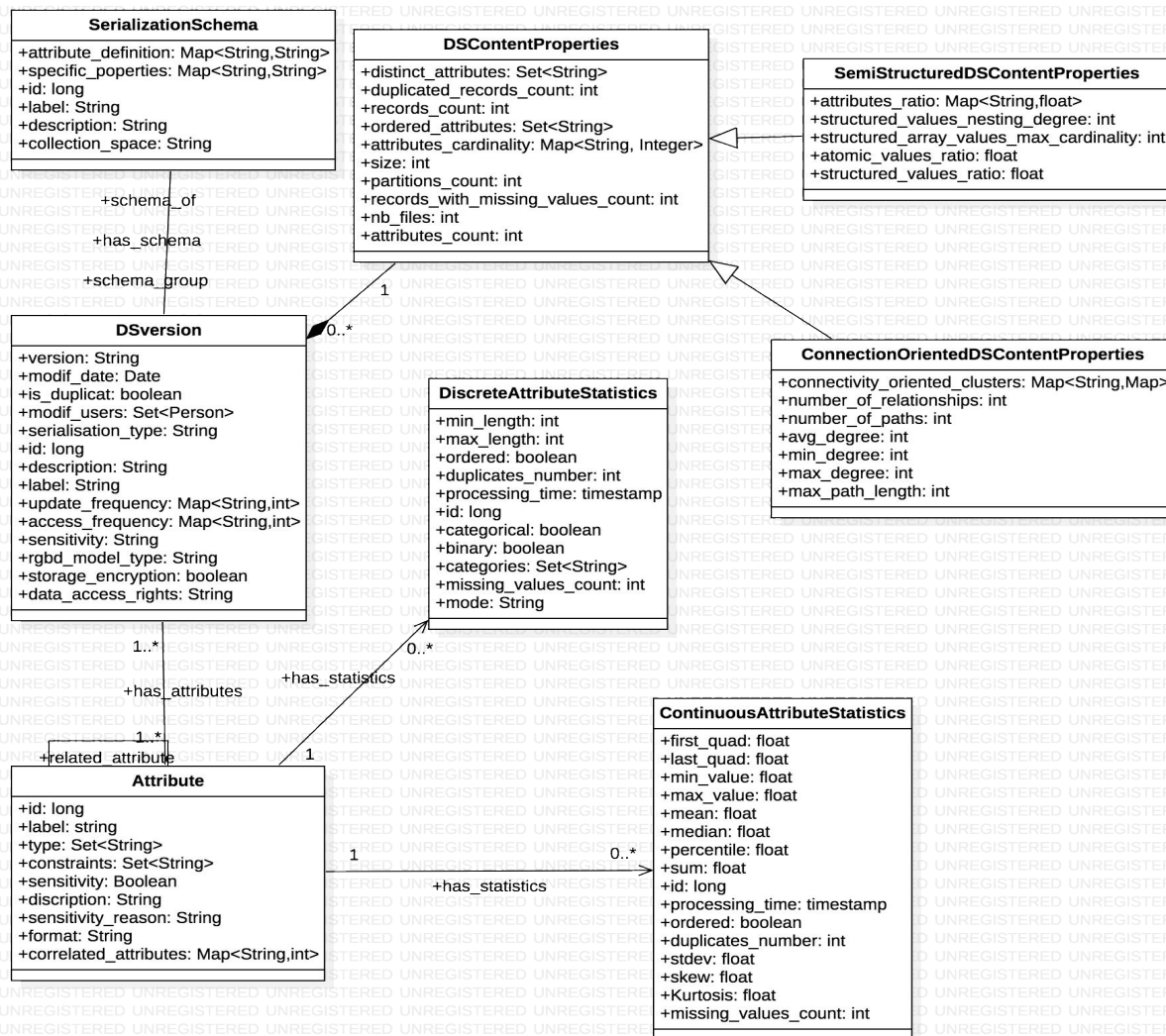
Figure 3.3 Diagramme de classe pour les métadonnées : statistiques sur les ensembles des données
