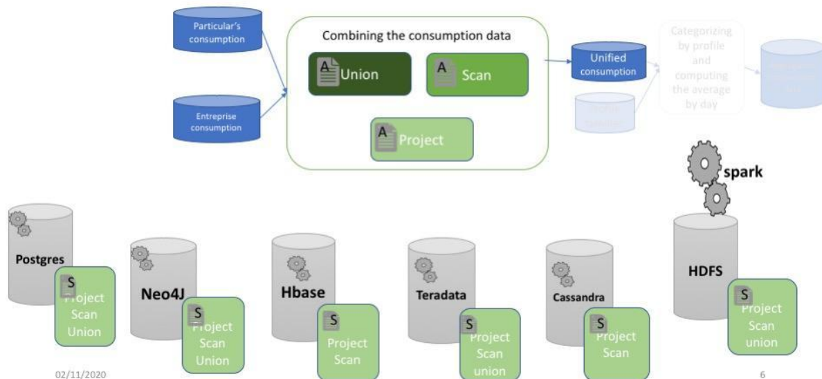
Figure 4.4 Exemple de métadonnées utilisées dans l'algorithme de construction de l'espace de recherche
