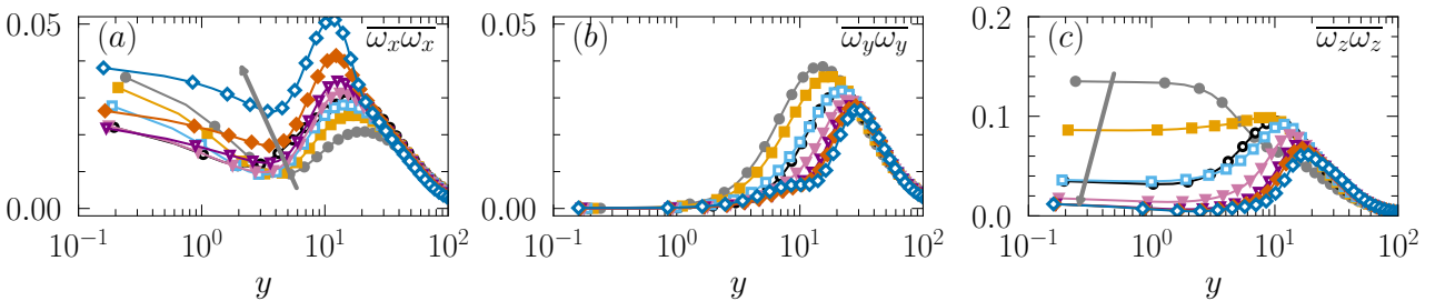
Figure 5: Profils d’ensrophie moyens pour les cas non contrôlés et contrôlés. Se référer à la figure 1 pour les symboles correspondant aux différents cas. Reproduit d’Umair & Tardu [14] avec l’autorisation de CUP.
