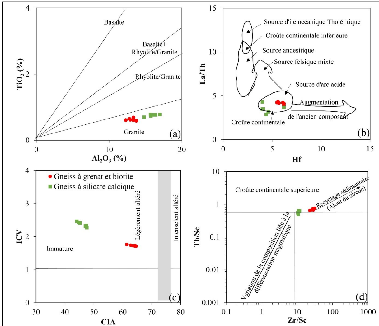
Figure 44. (a) Diagramme TiO_2 en fonction de Al_2O_3 (Ekosse, 2001); (b) Diagramme La/Th en fonction de Hf fonction de Zr/Sc (McLennan et al., 1993); (c) diagramme IVC en fonction de CIA (Nesbitt et Young, 1982); (d) Diagramme Th/Sc en fonction de Zr/Sc (McLennan et al., 1990).
