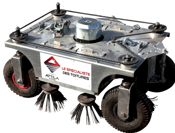
Figure 1.2: Prototype du robot : ATTILA.
