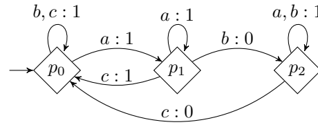
(d) A parity automaton recognising L with only 3 states .
