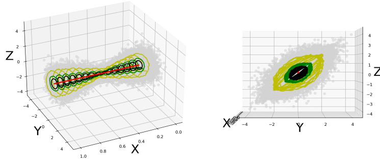
Figure 1.3: Ejemplo de regresión cuantílica univariante; con X e \mathbf{Y} = (Y, Z) como en (1.26). El número de puntos observados es n = 7,000 . Los contornos cuantiles para \tau = 0.2, 0.4, 0.8 están representados en negro ( \tau = 0.2 ), verde ( \tau = 0.4 ) y amarillo ( \tau = 0.8 ). El centro viene representado en rojo.
