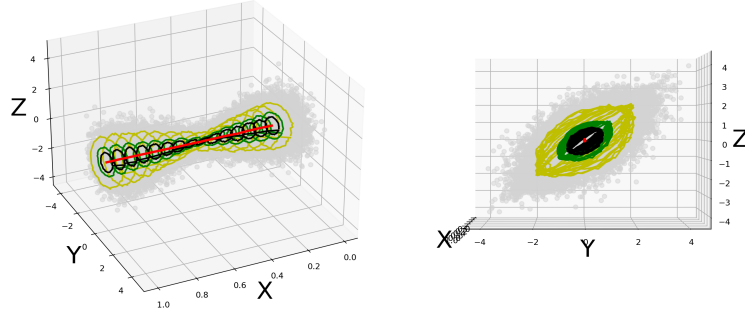
Figure 1.3: Exemple de régression quantile univariée; avec X et \mathbf{Y} = (Y, Z) comme dans (1.26). Le nombre de points observés est n = 7000 . Les contours du quantile pour \tau = 0, 2, 4, 6, 8 sont représentés en noir ( \tau = 0, 2 ), vert ( \tau = 0, 4 ) et jaune ( \tau = 0, 8 ). Le centre est représenté en rouge.
