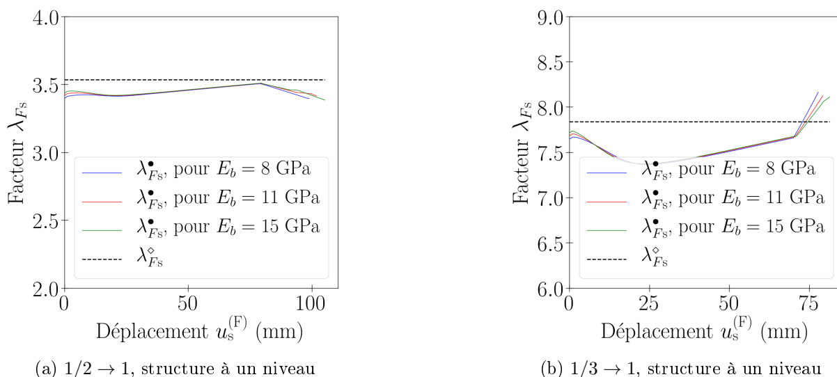
FIGURE 4.26 – Modification du module d'Young E_b du bois, facteur \lambda_{F_s}
