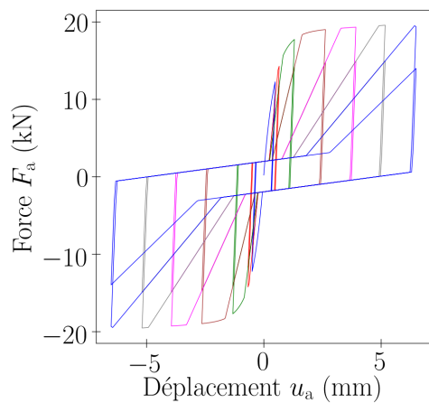
(c) courbe force déplacement Saws , échelle 1/2
