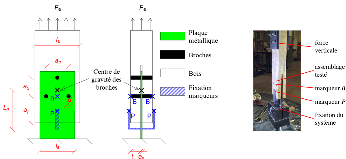
FIGURE 2.5 – Montage des essais axiaux sur assemblages
