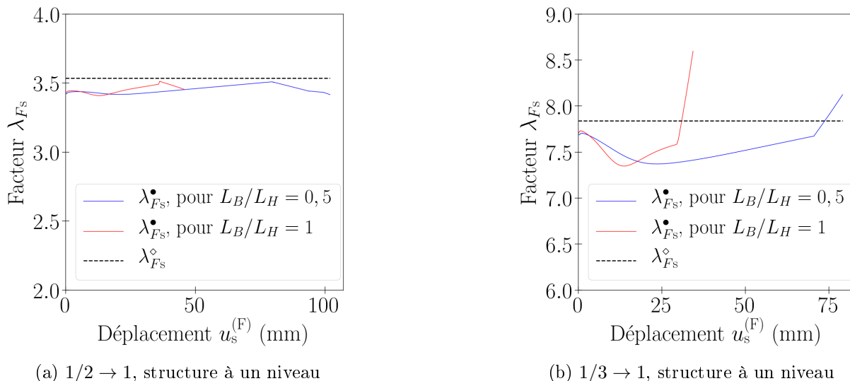
FIGURE 4.25 – Modification du rapport L_B/L_H (en conservant L_H ), facteur \lambda_{F_s}
