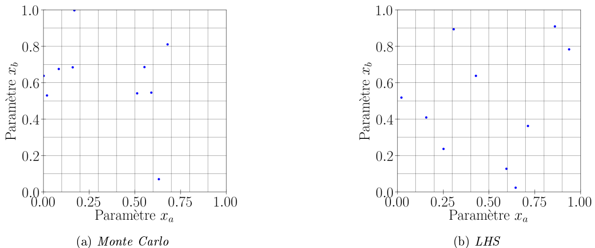
FIGURE 4.33 – Exemples de plans d'expériences Monte Carlo et LHS
