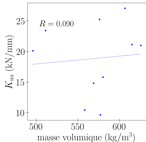
(f) masse volumique et K_{ua} , échelle 1/3
