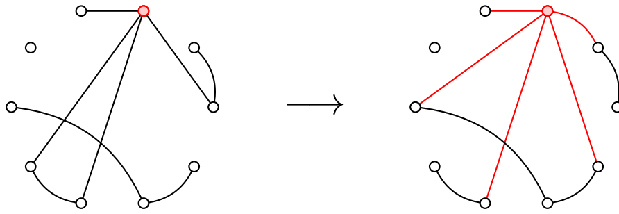
Figure 1.14 – Illustration d'une transition du graphe aléatoire inhomogène dynamique avec mise-à-jour par sommets. Le sommet rouge à gauche est celui choisi pour être mis à jour. Les arêtes rouges à droite sont les nouvelles arêtes formées.
