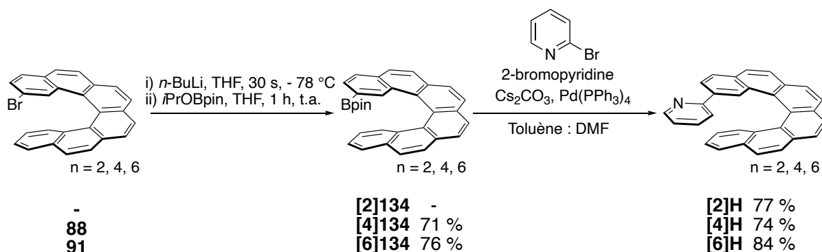
Figure 107. Synthèse des dérivés 2-([n]héliçèn-2-yl)-2-pyridine [n]H .
