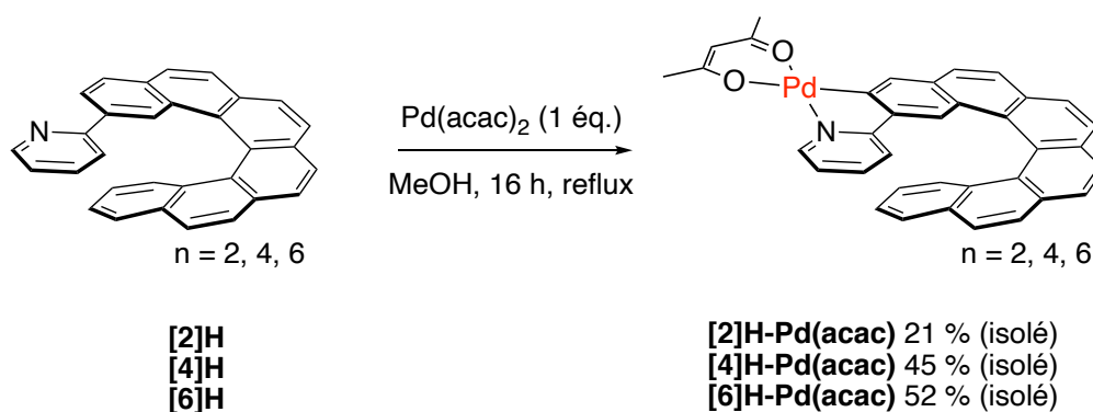
Figure 108. Synthèse des complexes précurseurs [n]H-Pd(acac) .
