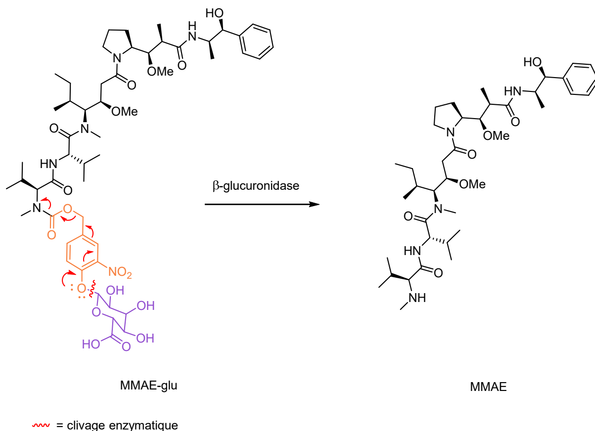
Figure 3 – Evolution de la prodrogue MMAE-glu sous l'action de la \beta -glucuronidase.
