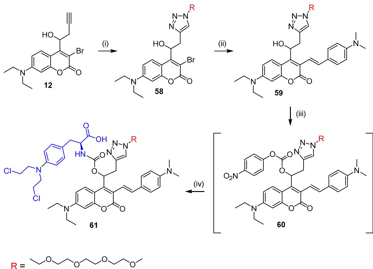
Schéma 51 – Synthèse de l'analogue photoactivable 61 ; (i) R-N_3 , acide ascorbique, tris(3-hydroxypropyltriazyloyméthyl)amine, Cu(CH_3CN)_4PF_6 , CH_2Cl_2 , TA, 22 h, 38 % ; (ii) 9 , K_2CO_3 , Pd(PPh_3)_4 , H_2O/DME (1:3), chauffage au micro-onde à 105 °C, 1 h 20, 46 % ; (iii) carbonate de bis-(4-nitrophényle), DIPEA, DMF, TA, 22 h ; (iv) melphalan, DIPEA, DMAP, DMF, TA, 4 h, 47 % sur les deux étapes.
