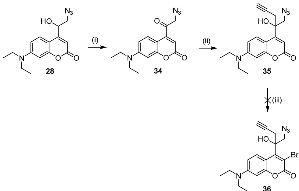
Schéma 36 - Première approche vers une coumarine trifonctionnalisée par un azoture, un alcyne terminal et un alcool. (i) Périodinate de Dess-Martin, \text{CH}_2\text{Cl}_2 , 0^\circ\text{C} à TA, 4 h, 56 % ; (ii) bromure de propargylzinc, THF, 0^\circ\text{C} à TA, 1 h 30, 78 % ; (iii) NBS, acétate d'ammonium, MeCN, TA, 40 min.
