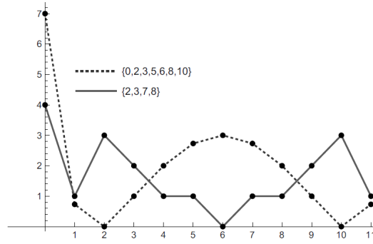
Figure 9: La DFT (en module) d'une mélodie et son accompagnement chez Bartok (figure extraite de [4]).
