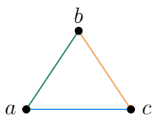
Graphe G initial.
