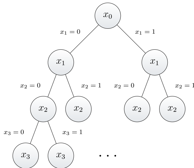
FIGURE 1.11 – Structure d'arbre d'énumération.
