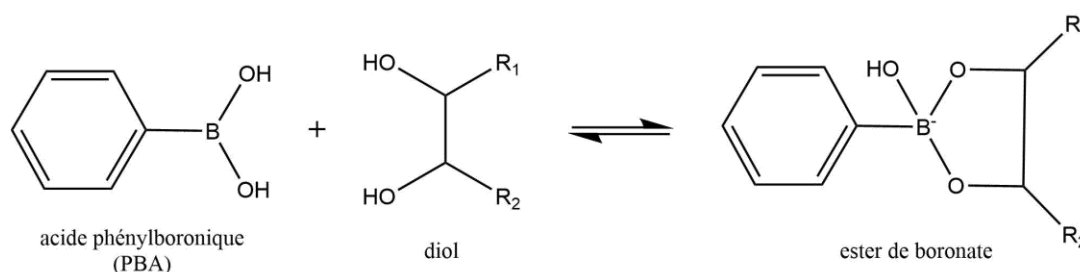
Figure 13 : Formation d'ester de boronate via la complexation entre un acide boronique et un diol.
