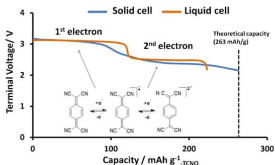
FIGURE 1.12 – réaction d’oxydo-réduction de la TCNQ, potentiel et capacité obtenus en batterie liquide et possibilité de modifications des ses propriétés[55]
