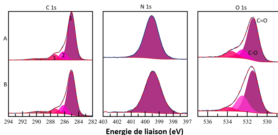
FIGURE 3.4 – Spectres XPS C 1s, N 1s et O 1s de la DAAQ (A) et du mélange de la 2,6-diamino-anthraquinone avec l'argyrodite \text{Li}_6\text{PS}_5\text{Cl} (B)
