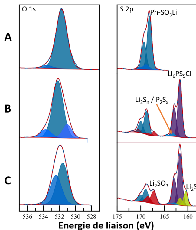
FIGURE 3.20 – Spectres XPS O 1s et S 2p du Li 4 -p-DHBDS (A), du mélange Li 4 -p-DHBDS / Argyrodite (B) et de l'électrode après cyclage (C)
