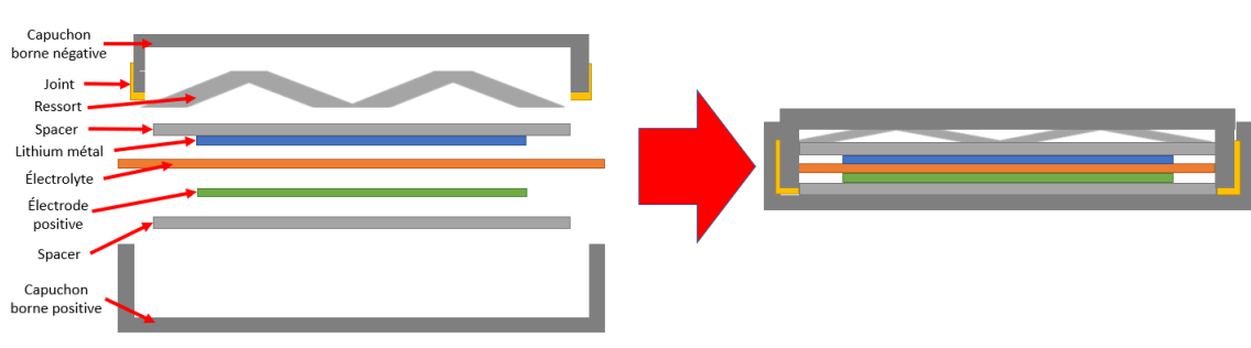
FIGURE 2.3 – Schéma du montage des batteries en pile bouton
