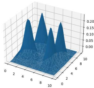
(a) Vraie fonction
