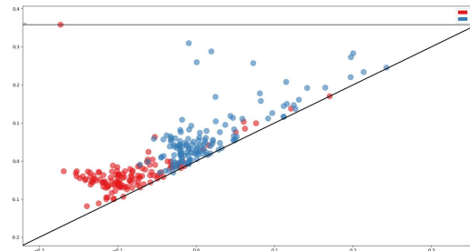
(d) Diagramme de persistance correspondant
