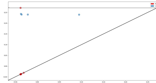
(b) Diagramme de persistance correspondant
