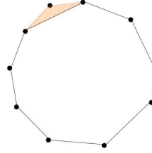
(b) Complexe de Čech correspondant
