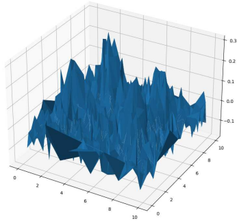
(c) Fonction bruitée
