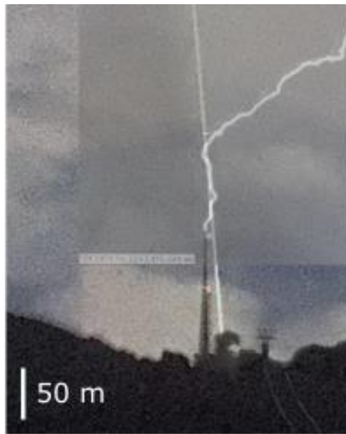
Figure 6 : Image capturée par une caméra rapide de la propagation d'un des éclairs observés en présence de filaments laser. Une photo prise du même angle de vue que la caméra et montrant la trajectoire du laser y est superposée, mettant en évidence le phénomène de guidage.
