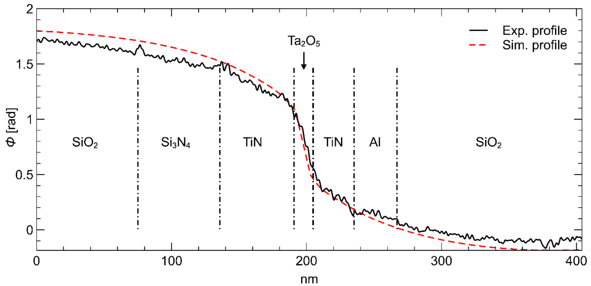
Figure 6.3 : Profils extraits des images de phase expérimentales et simulées le long des flèches noires sur les images de phase Figure 6.2b, c.
