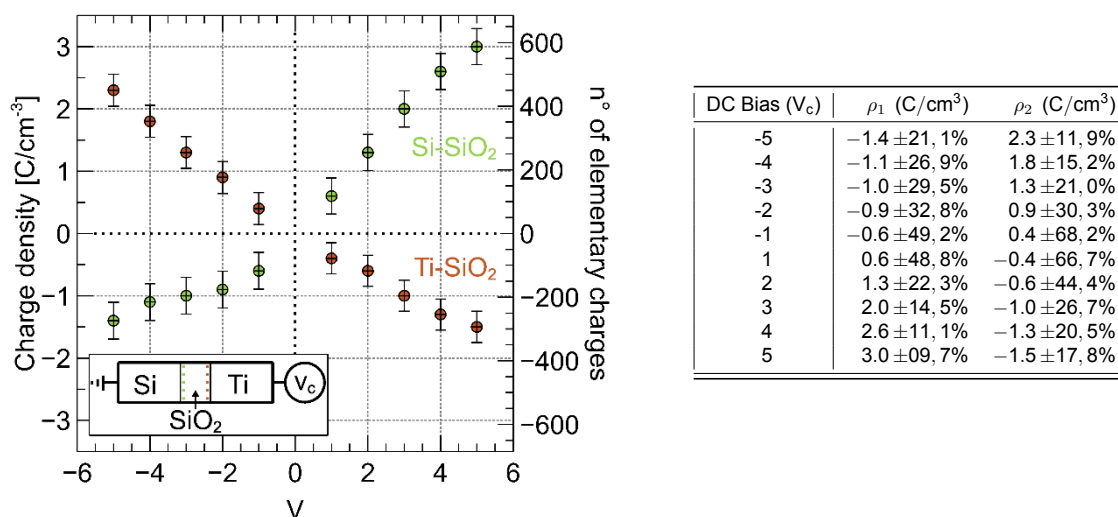
Figure 4.8 : Charge diélectrique aux interfaces Si-SiO 2 ( \rho_1 ) et SiO 2 -Ti ( \rho_2 ) en fonction de la polarisation appliquée. Les charges par unité de volume sont représentées sur l'axe gauche. Le nombre de charges élémentaires contenues dans la région analysée du dispositif expérimental est représenté par les axes de droite. Le tableau des données est présenté avec l'incertitude sur la droite.
