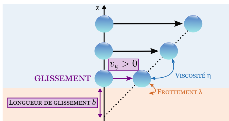
Figure 8.14: Schéma de la condition limite de glissement.
