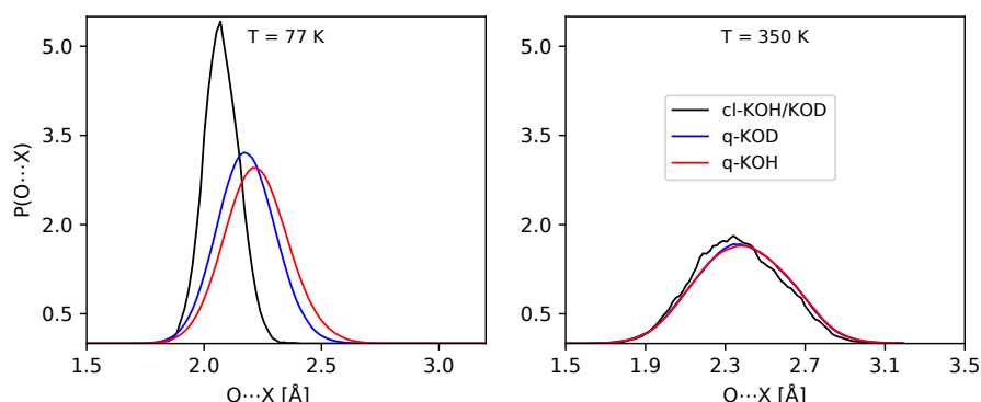
Figure IV: Distribution de probabilité de la longueur O...X obtenue par des simulations ab initio classiques ( cl -KOH/D) et PIMD de l'hydroxide de potassium hydrogéné ( q -KOH) et deutéré ( q -KOD).
