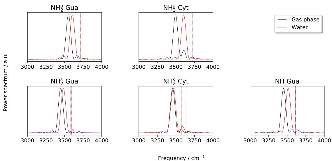
Figure X: Spectres QCT des vibrations du stretching de NH interbase en phase gazeuse et dG-dC solvaté à l'aide d'AMOEBABIO18. Les valeurs harmoniques correspondantes sont indiquées sous forme de lignes pointillées verticales.
