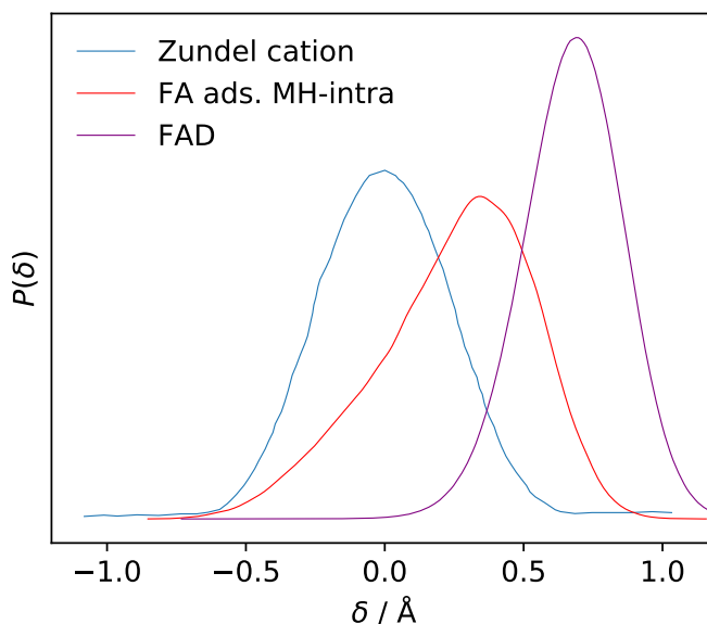
Figure VII: Distribution de probabilité à température 100 K de la coordonnée du "proton sharing" \delta dans le cation zundel (Shran et al. [191], Figure 4, courbe à 2.4 \text{ \AA} ), l'acide formique adsorbé sur la surface d'anatase (101) et le dimère d'acide formique en utilisant la PES de Qu et al. [190].
