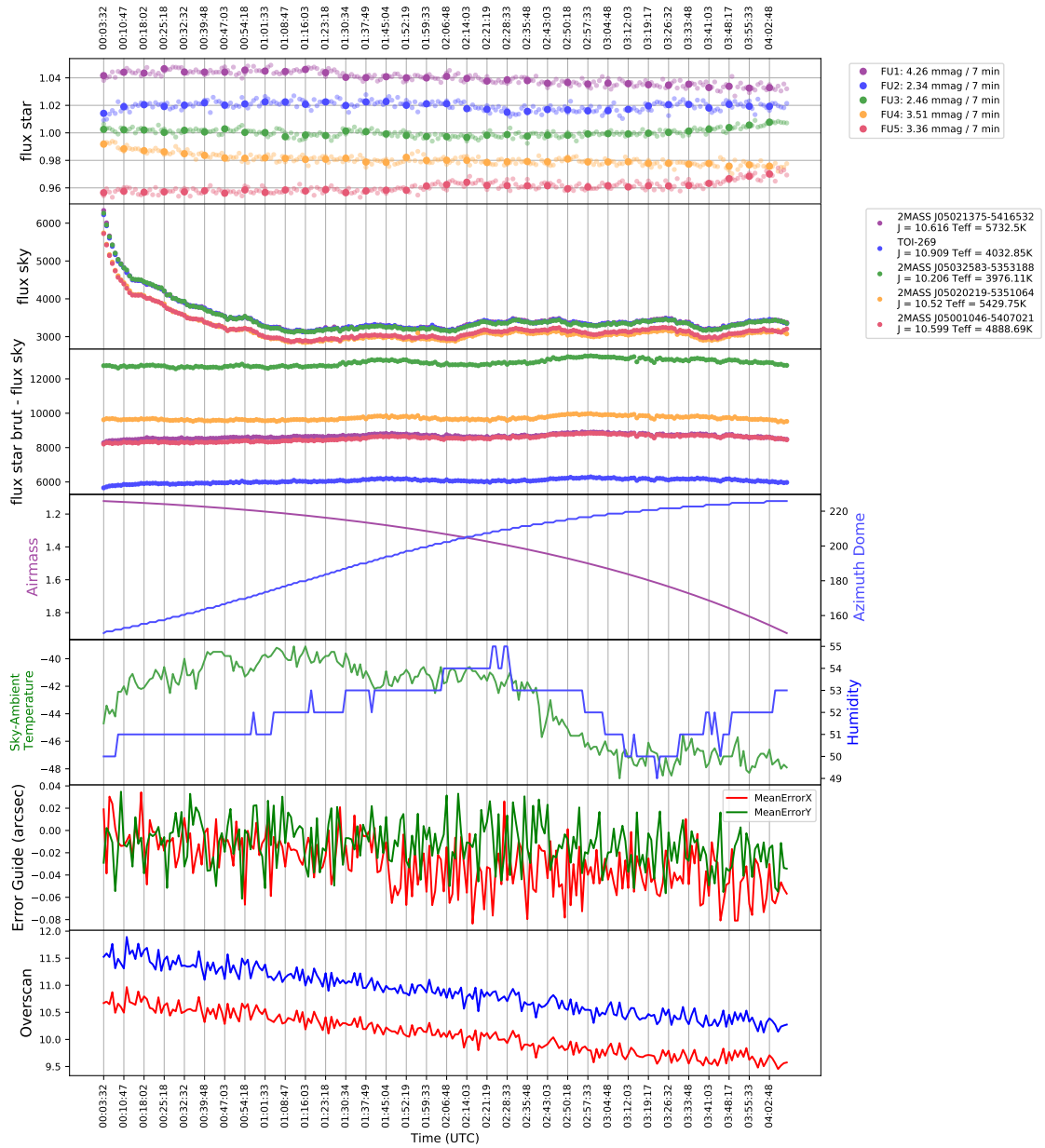
2020-03-01 Tel1 TOI-269_W_2019-12-18.fits
