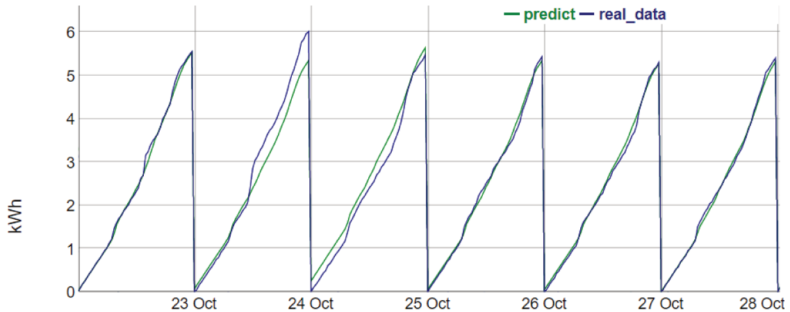
FIGURE 4.54 – Exemple de prévision à (J+1) par le modèle KWF de la série temporelle de l'énergie journalière consommée du ménage M_9 pour la période allant de 22 à 28 octobre 2022. La courbe en bleu représente la consommation réelle tandis que la courbe en vert représente les prévisions. Les erreurs de prévision NMAE et NRMSE des données d'énergie journalière consommée de ce ménage sont respectivement 0,09 et 0,14.
