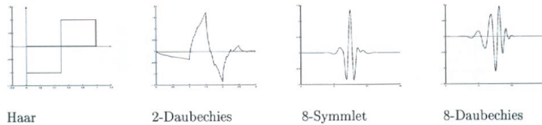
FIGURE 7.35 – Exemples d'ondelettes [Source (CHARLES et al., 2004)].
