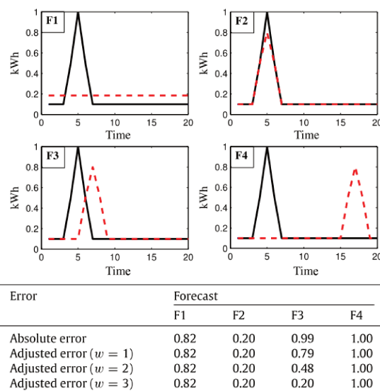
FIGURE 3.4 – Les quatre graphiques représentant les différentes prévisions F_1, F_2, F_3 et F_4 (ligne en pointillés rouge) d’une courbe de charge (ligne noire continue) ainsi que les erreurs absolues ( w=0 ) et ajustées ( w=1,2 et 3 ) de la p-norme [source (HABEN, WARD et al., 2014)].
