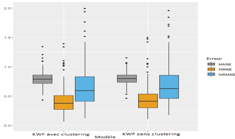
FIGURE 4.26 – Les boîtes à moustaches des erreurs de prédiction par le modèle KWF et le modèle KWF avec clustering des ménages thermosensibles.
