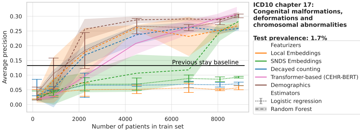
Fig. C.27. ICD10 chapter 17
