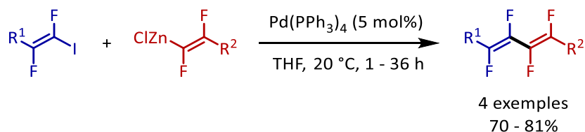
Schéma 104. Préparation de diènes fluorés de Sauvêtre.
