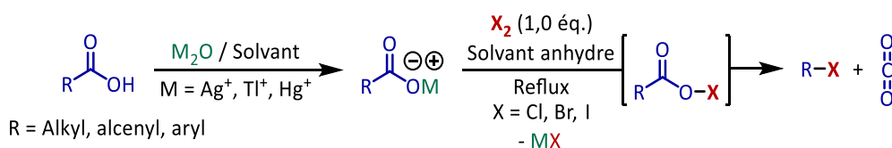
Schéma 118. Réaction générale de Hunsdiecker.
