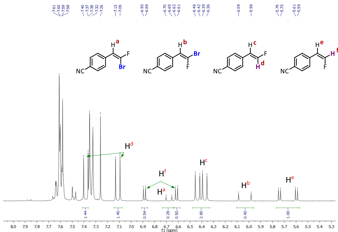
Figure 29. Analyse RMN 1 H de l'expérience d'inhibition de radicaux avec le BHT.
