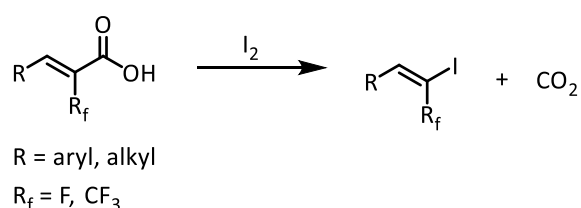
Schéma 134. Objectif du deuxième projet.
