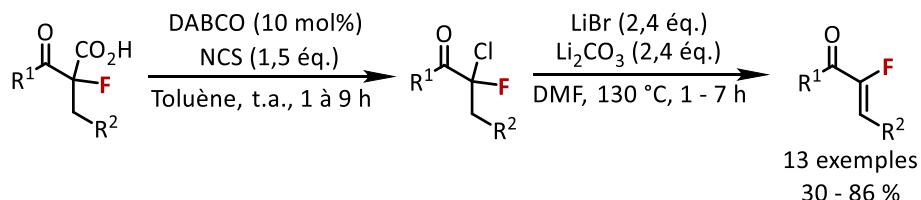
Schéma 16. Synthèse d' \alpha -fluorénones par élimination du chlore.
