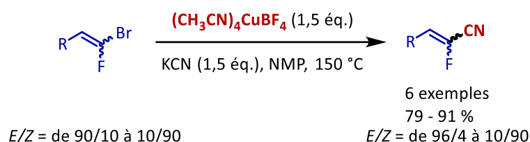
Schéma 99. Cyanation de gem -bromofluoroalcènes développée par Rolando.
