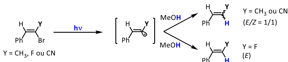
Schéma 49: Photolyse de \beta -bromostyrènes \beta -substitués.
