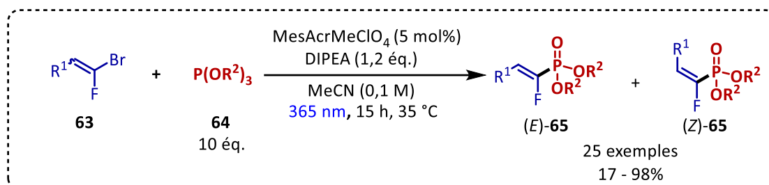
Schéma 84. Nouvelle méthode de synthèse d' \alpha -fluorovinylphosphonates par catalyse photoredox développée pendant cette thèse.
