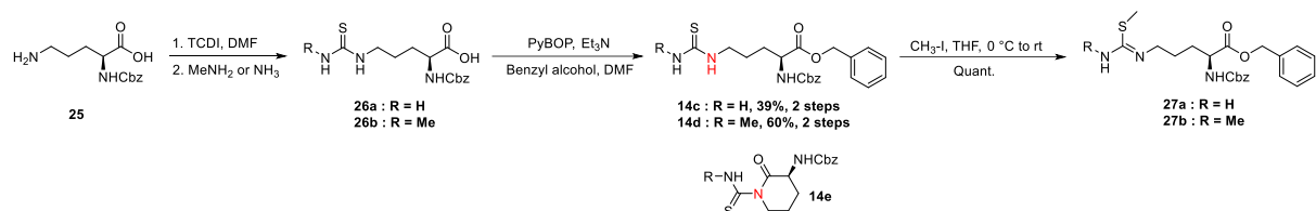
Schéma 8: Synthèse des isothiourées
