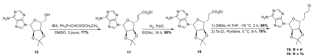
Schéma 3: Synthèse du nucléoside tosylé permettant l'accès aux deux amines
