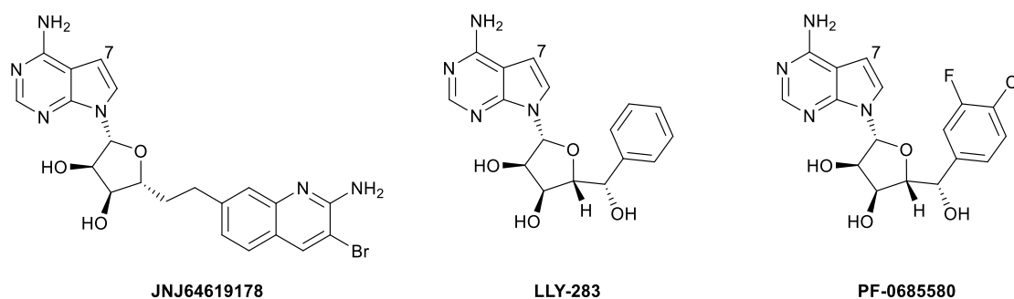
Figure 29: Les inhibiteurs analogues du SAM en essais cliniques
