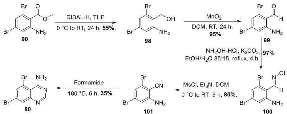
Schéma 24: Voie alternative pour la synthèse du corps central
