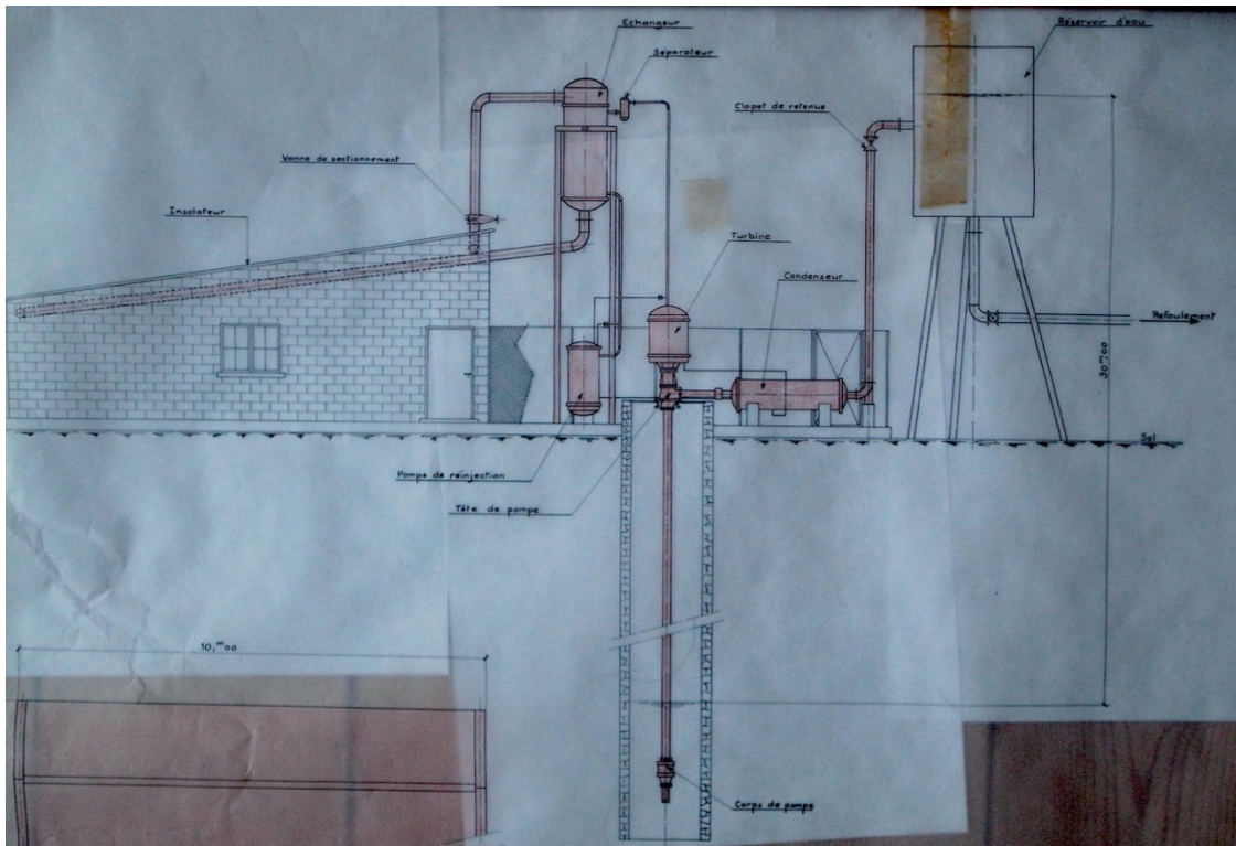
Figure 6 : une version d'ITTEC sur puits. Nous constatons que les capteurs abritent un bâtiment. Plan 21437, 15 avril 1965, archives privées fonds usine Mengin.
