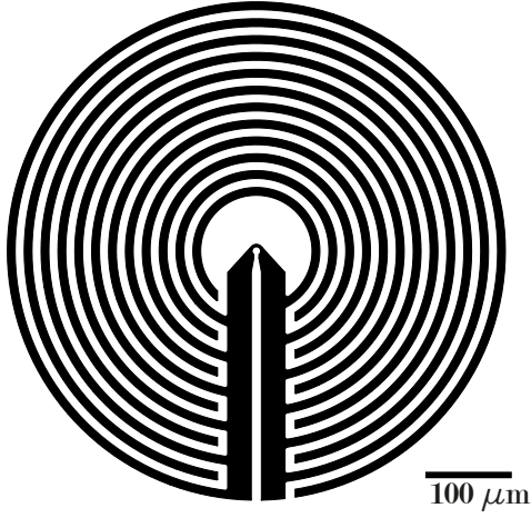
Figure 1.2: Géométrie du résonateur. La boucle inductive au centre a un rayon de 5\text{ }\mu\text{m} , la zone à l'intérieur de cette boucle est l'espace où est inséré l'échantillon.
