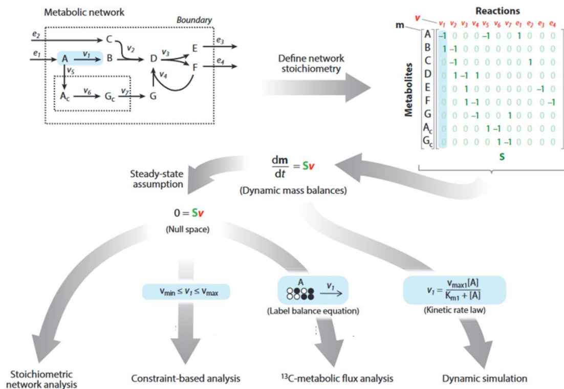
Figure 1.36 : Approches de modélisation métabolique. Illustration adaptée de Clark et al, 2020. Abréviations : A : concentration du métabolite A ; K_m : constante de liaison de Michaelis ; v_{\max 1} : vitesse maximale de la réaction 1
