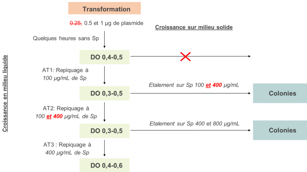
Figure III-6 : Etapes de sélection et de criblage optimisées afin de délétér des gènes cibles chez la souche BerOc1. Sp: spectinomycine (antibiotique de sélection des cellules transformées).
