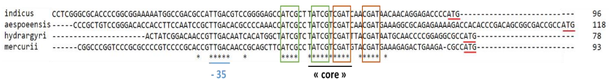
Figure V-8 : Alignement multiple des régions intergéniques en amont du gène arsR chez des souches méthylantes. Les ATG sont soulignés en rouge. La boîte -35 est conservée et soulignée en bleu. Les identités sont marquées par un astérisque (*). Les motifs répétés dans le sens direct sont encadrés en vert et ceux répétés dans le sens inverse sont encadrés en orange. La séquence « core » (10 nucléotides) est soulignée en noir.
