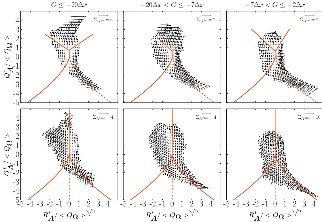
Figure C.12. CMT du LEE dans la région éloignée (colonne de gauche), intermédiaire (colonne du milieu) et proche (colonne de droite) dans le plan de phase (R_A^*, Q_A^*) pour le cas multiphasique avec \phi_\ell = 0.10 . Les termes des équations d'évolution présentées correspondent à \Pi^{local} : pression locale contribution Hessienne (rangée du haut); et \Pi^{nonlocal} : contribution Hessienne de pression non locale (rangée du bas). L'échelle du vecteur de chaque terme est calculée en fonction de la longueur moyenne du vecteur \left( \overline{X_{\langle \dot{R}^*, \dot{Q}^* \rangle}} = \left\| \sqrt{(\dot{R}_A^*)^2 + (\dot{Q}_A^*)^2} \right\| \right) et son écart type correspondant \left( \sigma_{\langle \dot{R}^*, \dot{Q}^* \rangle} \right) comme suit : \Sigma_{term} = \overline{X_{\langle \dot{R}^*, \dot{Q}^* \rangle}} + 3\sigma_{\langle \dot{R}^*, \dot{Q}^* \rangle} .
