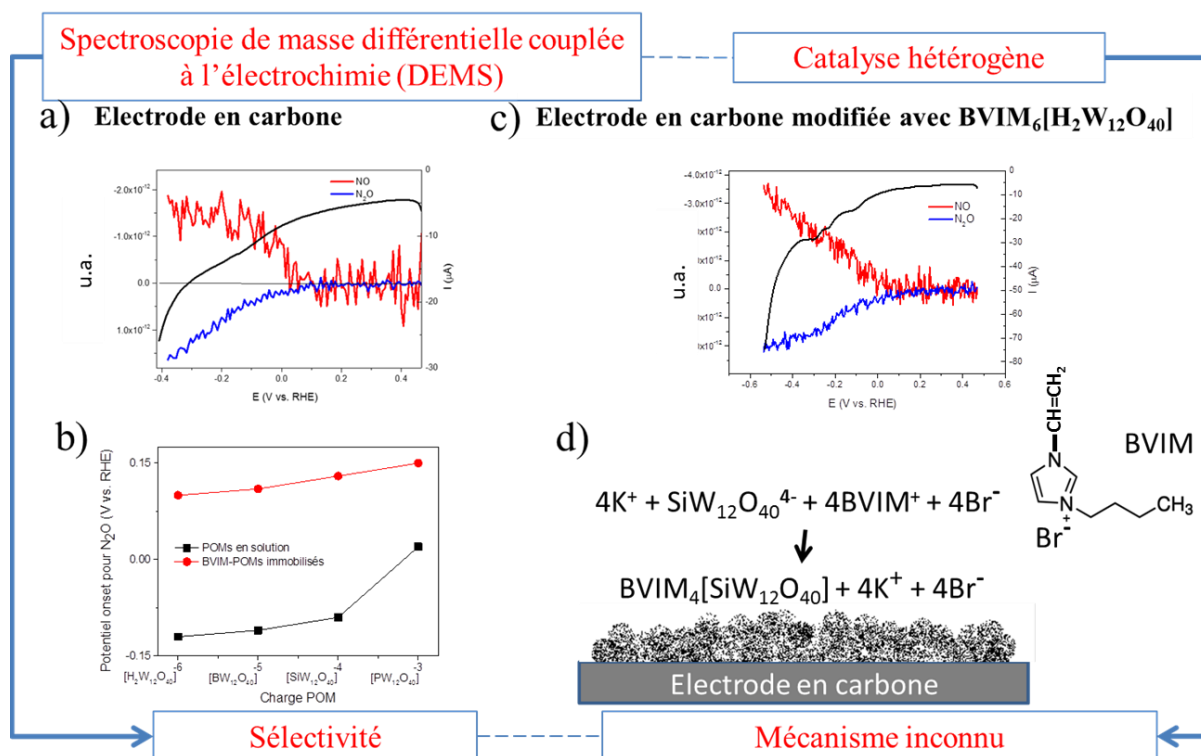
Figure 3. a) Analyse DEMS de la réduction des nitrites au niveau d'une électrode en carbone ; b) Analyse DEMS de la réduction des nitrites sur une électrode de carbone modifiée avec l'hybride BVIM 6 [H 2 W 12 O 40 ] immobilisé ; c) Potentiel d'apparition de N 2 O obtenu à partir d'une analyse DEMS à différentes électrodes ; d) Équation de la réaction chimique entre le POM K 4 [SiW 12 O 40 ] et le liquide ionique le bromure de 1-butyl-3-vinyl imidazolium (BVIM) formant le composé insoluble BVIM 4 [SiW 12 O 40 ] qui est ensuite immobilisé sur une électrode de carbone. (BVIM = 1-butyl-3-vinyl imidazolium).
