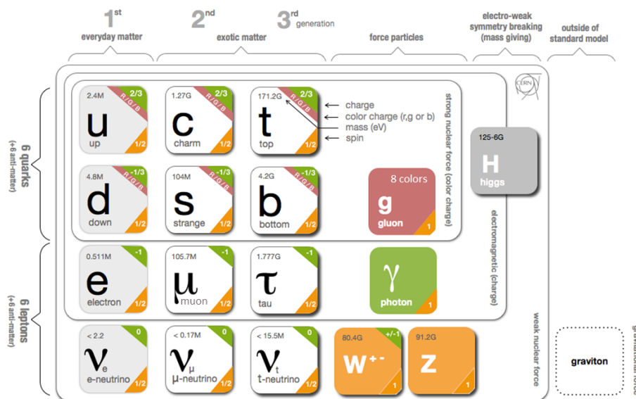
Figure K.1 – Zoologie schématisée de l'ensemble des particules élémentaires du Modèle Standard (et gravitation), après brisure spontanée de la symétrie électrofaible.
