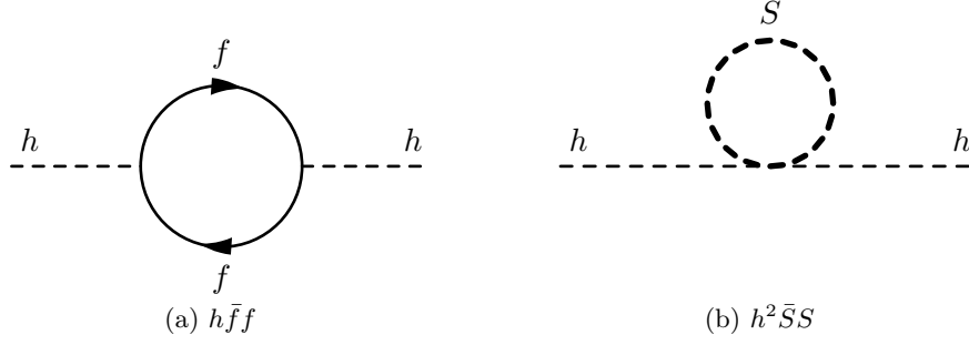
Figure K.2 – Corrections à la masse du Higgs au carré m_{h,\text{phys}}^2 , dues aux (a) fermions de Dirac f [anti-particule \bar{f} ], et (b) aux champs scalaires complexes S [anti-particule \bar{S} ].
