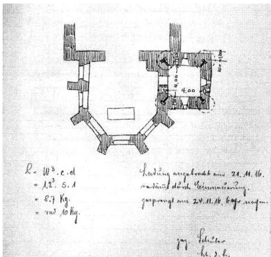
Figure 7 - Esquisse et calcul pour la destruction du clocher d'Ammertzwiller.
